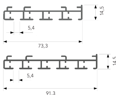
skenprofil 4 & 5 spår
