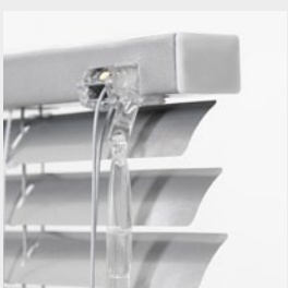
Triangulär vridstång – ett estetiskt tilltalande alternativ till den sexkantiga som är standard (Embla)
